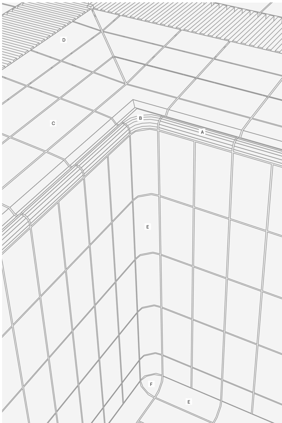
A Ref. 954 / Ref. 953 Borde sport / finlandés 12 x 24,5 x 2,6 cm
